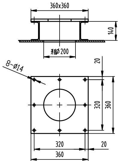
槽钢架与安装底板安装示意图
